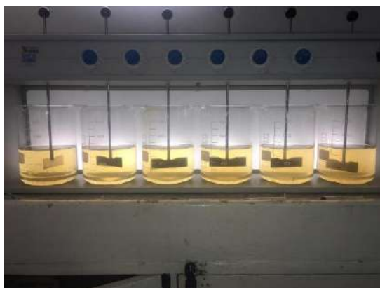
Figura 2. Fotografía que presenta la prueba de jarras para la mezcla coagulante químico-natural.
