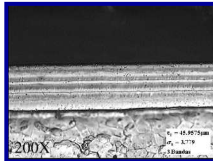
Figura 1. Recubrimiento químico Ni-P-Mo sobre acero al carbono. Microscopía Electrónica de Barrido (200 X) [3]
