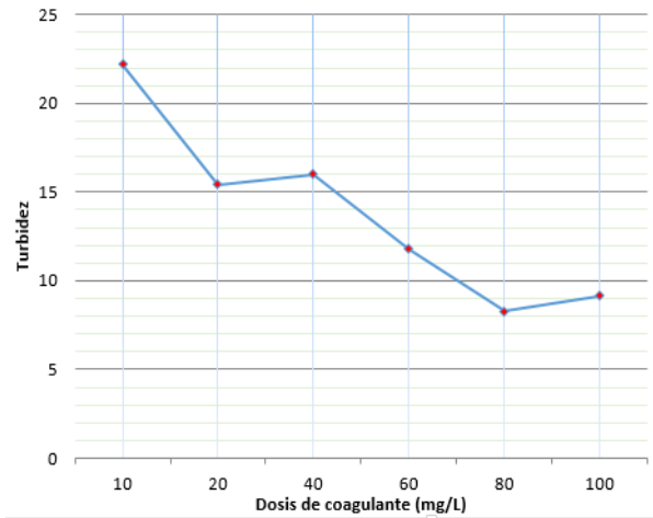
Figura 2. Turbidez final del agua después de la prueba de jarras vs Dosis del coagulante químico.
